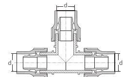
KİLİTLİ BAĞLANTI TE LOCK TYPE TEE
