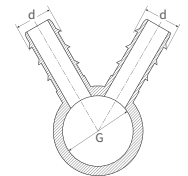
KURTAĞZI ÇOKLU DAĞITIM NİPELİ BARBED MULTICOUPLING NIPPLE
