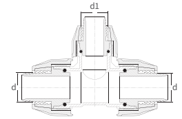
REDÜKSİYON TE REDUCING TEE
