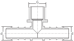
KURTAĞZI - ERKEK TE BARBED - MALE TEE
