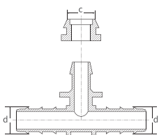
KURTAĞZI - GROMMET TE BARBED - GROMMET TEE
