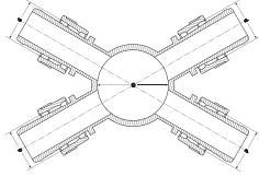
YÜZÜKLÜ YASSI ÇOKLU DAĞITIM NİPELİ TAPE (WITH RING) MULTICOUPLING NIPPLE
