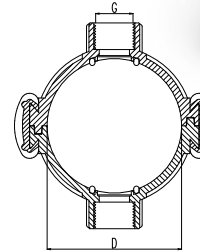
PRİZ KOLYE ÇİFT ÇIKIŞLI GEÇMELİ DOUBLE ENDED CLAMP SADDLE WITH SLIDE
