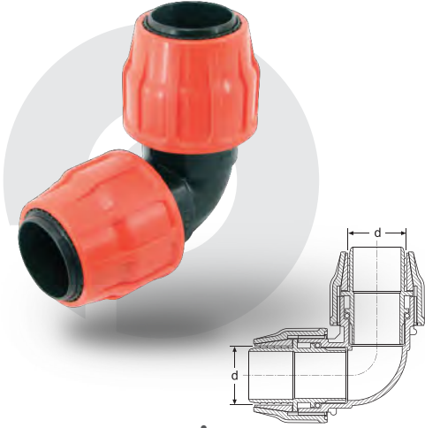
LAYFLAT DİRSEK LAYFLAT ELBOW
