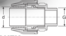
LAYFLAT ERKEK LAYFLAT MALE ADAPTOR
