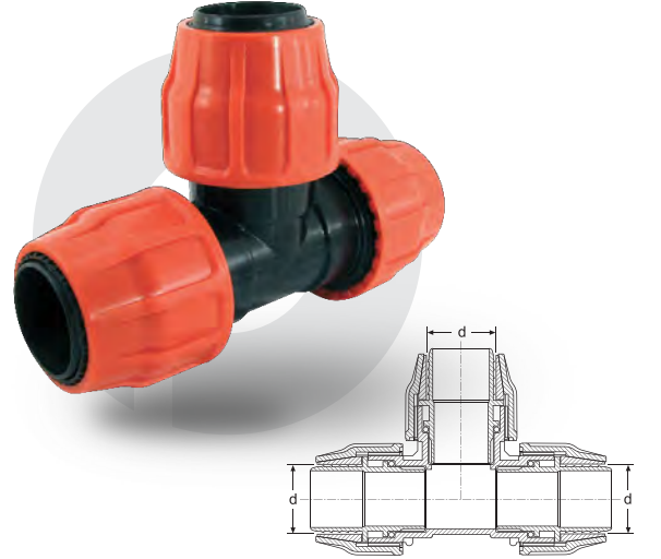
LAYFLAT TE LAYFLAT TEE
