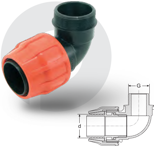
LAYFLAT ERKEK DİRSEK LAYFLAT MALE ELBOW
