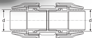
LAYFLAT MANŞON LAYFLAT COUPLING
