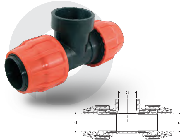
LAYFLAT DIŞİ TE LAYFLAT FEMALE TEE
