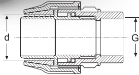
LAYFLAT DIŞI LAYFLAT FEMALE ADAPTOR
