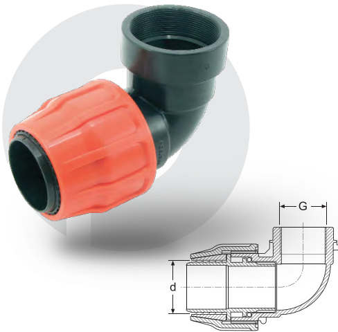
LAYFLAT DIŞİ DİRSEK LAYFLAT FEMALE ELBOW
