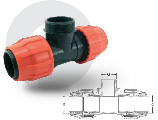
LAYFLAT ERKEK TE LAYFLAT MALE TEE
