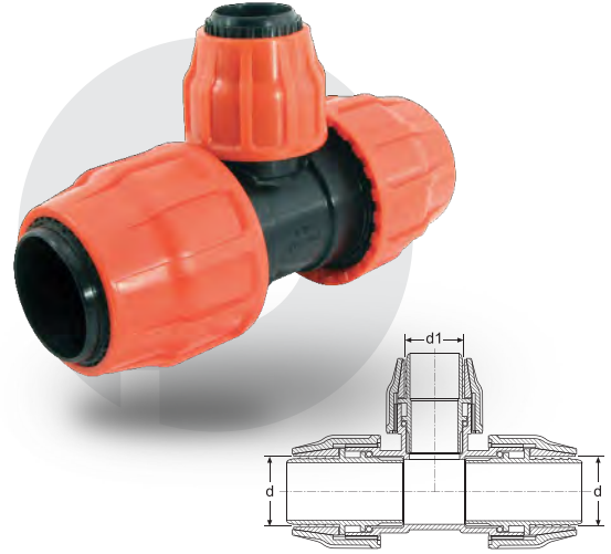
LAYFLAT REDÜKSİYON TE LAYFLAT REDUCING TEE
