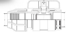
KÜRESEL VANA KABLİN - DIŞI BALL VALVE COUPLING - FEMALE
