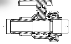
KÜRESEL VANA ERKEK - DIŞI BALL VALVE MALE - FEMALE
