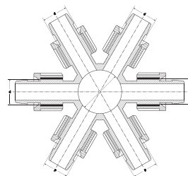
DAMLAMA ÇOKLU DAĞITIM NİPELİ DRIPLINE MULTICOUPLING NIPPLE
