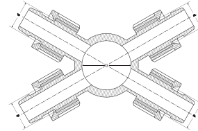
DAMLAMA ÇOKLU DAĞITIM NİPELİ DRIPLINE MULTICOUPLING NIPPLE
