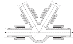
DAMLAMA ÇOKLU DAĞITIM NİPELİ DRIPLINE MULTICOUPLING NIPPLE
