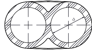
DAMLAMA GÖZLÜK KÖR TAPA FOLDING HOSE CONNECTOR END PLUG ЗАГЛУШКА КОЛЬЦЕВАЯ وصلة ( قابس ) نهاية لخرطوم الري بالتنقيط القابل للطي
