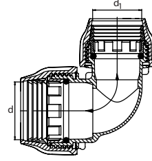
KABLİN REDÜKSİYON DİRSEK REDUCING ELBOW УГОЛ ПЕРЕХОДНОЙ
