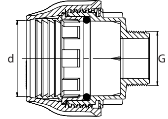
KABLİN ERKEK MALE ADAPTOR МУФТА С НАРУЖНОЙ РЕЗЬБОЙ
