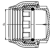
KABLİN KÖR TAPA END CAP ЗАГЛУШКА سدادة
