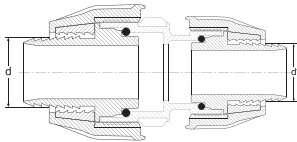
REDÜKSIYON MANŞON REDUCING COUPLING مصغرة
