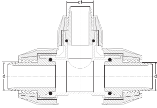
REDÜKSIYON TE REDUCING TEE تقسيم مصغري
