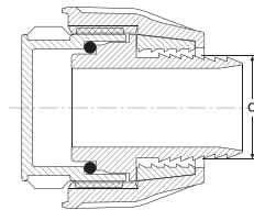
KÖR TAPA END CAP سدادة
