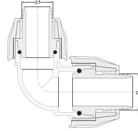
REDÜKSİYON DİRSEK REDUCING ELBOW عكس مصغرة
