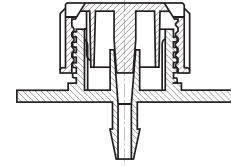
DEBİ AYARLI HAT ÜSTÜ DAMLATICI ON - LINE DRIPPERS КАПЕЛЬНИЦА С РЕГУЛИРОВКОЙ РАСХОДА قطرة
